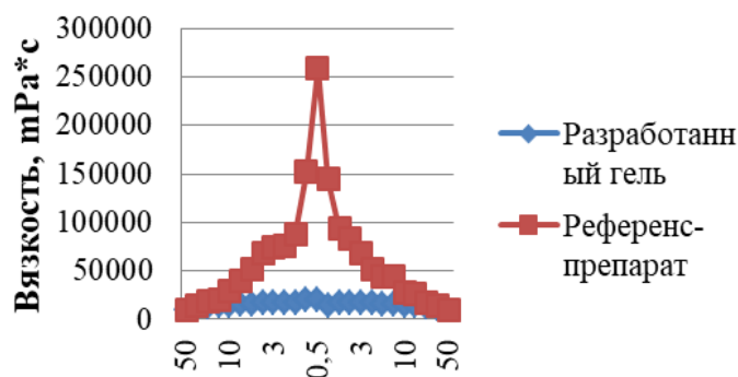
Рис. 2. Зависимость динамической вязкости от скорости вращения шпинделя при постоянной температуре 20° С
