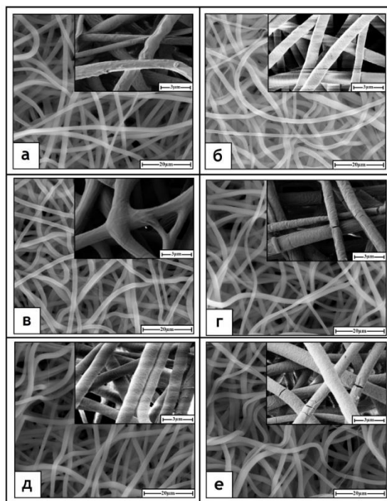
Рис. 1. СЭМ изображения PLLA скаффолдов, модифицированных в смеси различных газов: а – чистая атмосфера N_2 , б – смесь N_2 + He , в – смесь N_2 + Ne , г – смесь N_2 + Ar , д – смесь N_2 + Kr , е – смесь N_2 + Xe
