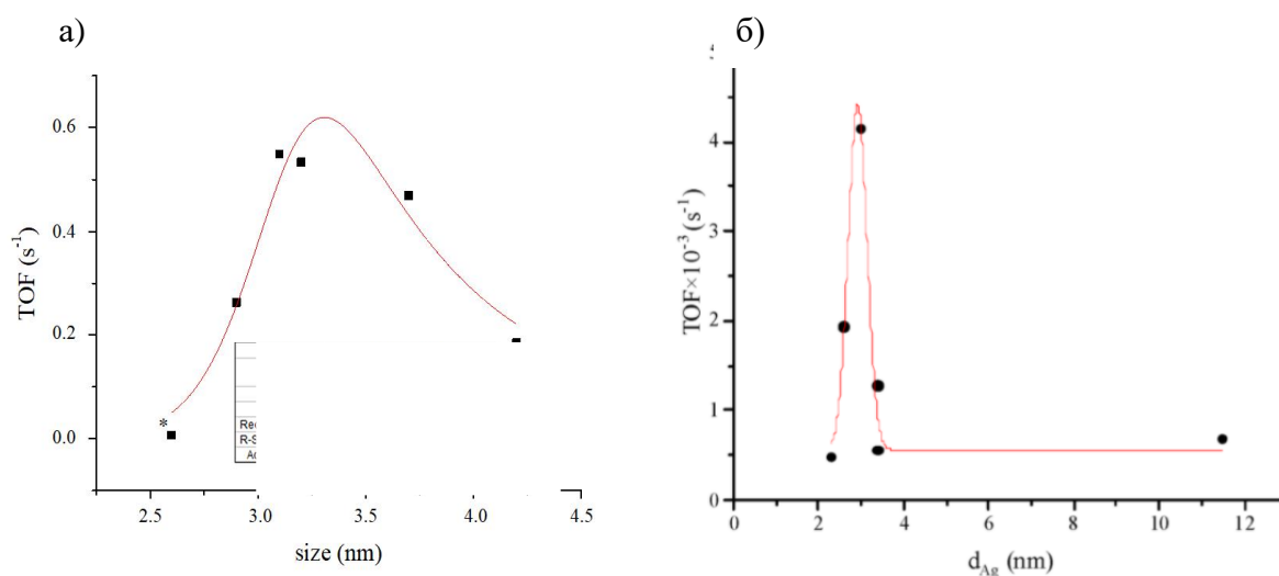
Рис. 1. Зависимость TOF от среднего размера наночастиц золота(а) и серебра(б)
