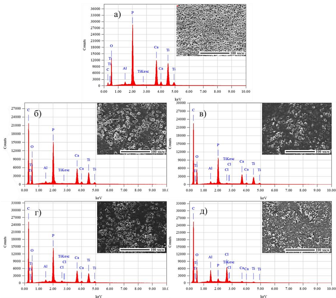
Рис. 1. СЭМ-изображения и энергетические спектры покрытий, сформированных методом МДО (а), МДО покрытия с поликапролактоном (б) и с добавлением хлорамфеникола: 5 масс. % (в), 15 масс. % (г), 25 масс. % (д)
