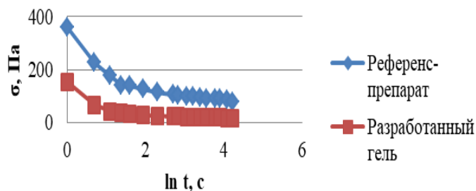
Рис. 1. Зависимость напряжения сопротивления структуры гелей от логарифма времени (по оси ординат – напряжение в Па, по оси абсцисс – \ln t , с.)
