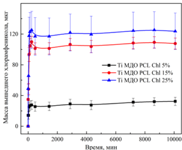
Рис. 2. Профили выхода хлорамфеникола из композиционных покрытий в течение 7 суток
