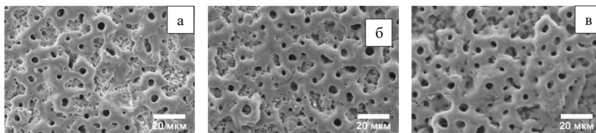
Рис. 1. СЭМ-изображение поверхности КФ-покрытия, сформированного методом МДО на поверхности титановой подложки (а), и гибридных покрытий с ПВП (б) и сополимером поли(молочной) и поли(гликолевой) кислот (в)
