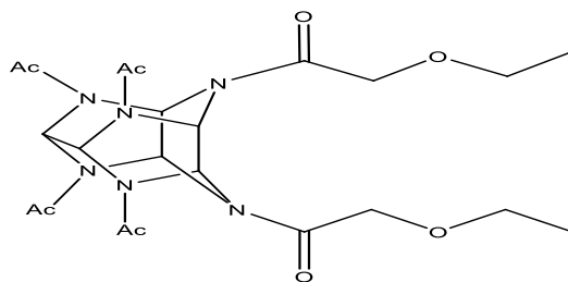
Рис. 3. Структурная формула 4,10-ди(этоксияцетил)-2,6,8,12-тетраацетил-2,4,6,8,10,12-гексаазатетрацикло[5,5,0,0 3,11 ,0 5,9 ]додекана (этовюрцин)
