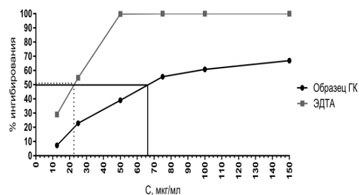
Рис. 2. Кинетические кривые реакции ингибирования гуминовыми кислотами образования комплекса феррозин- Fe^{2+}
