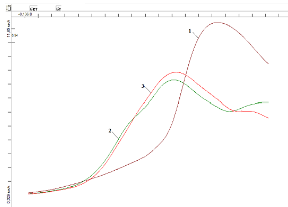
Рис. 4. Вольтамперограмма бетулина на графитовом электроде: 1 – фоновый электролит 0,1М NaOH, 2 –Аликвота БАД объемом 0.20 мл; 3 – добавка стандартного раствора бетулина, C_{\text{бет}} 575 \text{ мг/дм}^3 . W = 35 \text{ мВ/с} , t_{\text{нак}} = 25 \text{ с} , E_{\text{нак}} = -1,0 \text{ В} , дифференциальный режим регистрации.
