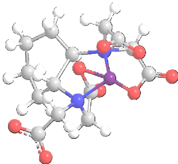
Рис. 1. Пространственная структура транс - 1, 2 - диаминоциклогексан-N,N,N',N' - тетрауксусной кислоты (ДЦТА) при формировании комплексов с Mn (Цикломанг) или 99m Tc (Циклотех), по данным квантово-химического моделирования.
