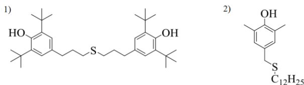
Рис. Структурные формулы: 1) бис-[3-(3,5-ди-трет-бутил-4-гидроксифенил)пропил]сульфид, 2) додецил(3,5-диметил-4-гидроксибензил)сульфид
