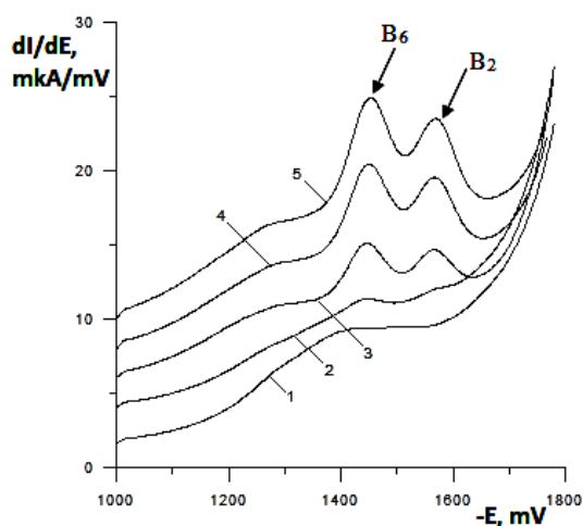
Рис. 2. Дифференциальные вольтамперограммы витамина В 2 и В 6 , полученных на графитовом (2) и новом модифицированном электроде (3-5), концентрация витаминов (С) мг/л: 4,0 (3), 10,0 (4), 16,0 (5). Фон: 0,1 М (NH 4 ) 2 SO 4 (1). Развёртка -0,5 до 1,8В, потенциал накопления -0,9В, скорость развёртки поляризующего напряжения - 35 мВ/с.
