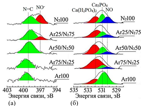
Рис. 1. XPS-спектры образцов: а – 1s спектр азота, б – 1s спектр кислорода
