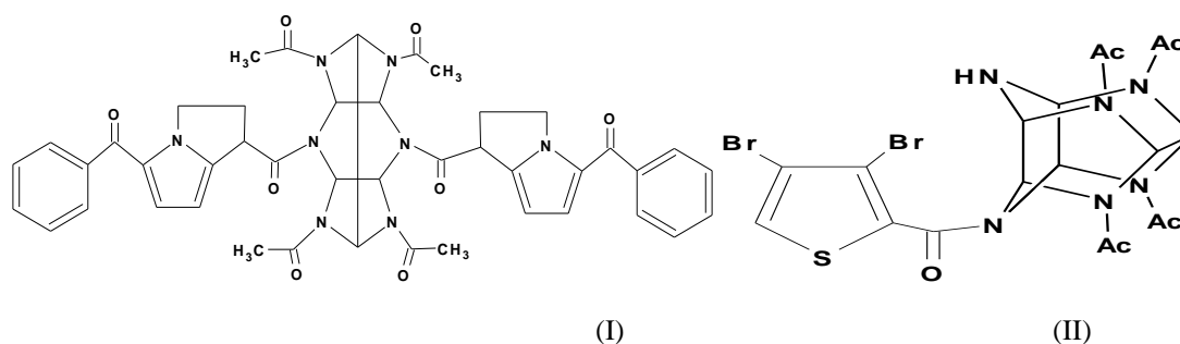
Рис. 2. Структурные формулы инновационных молекул.
