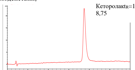
Рис. 1. Хроматограмма кеторолака ( k'_{\text{кеторолак}} = 6,50 ) при работе на фенильной стационарной фазе с подвижной фазой этилацетат – буфер триэтиламмония ацетата 20 мМ (99,9:0,1), подкисленный уксусной кислотой (40 мМ). Длина волны детектирования: \lambda = 275 нм; Температура термостата колонки: 30 °С; Объем вводимой пробы: 50 мкл. Объемная скорость потока: 1,0 мл/мин.
