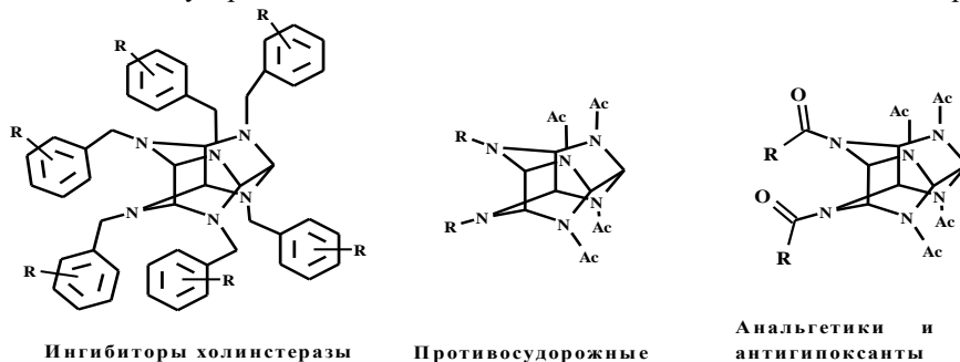
Рис. 1. Структурные формулы новых молекул-кандидатов
