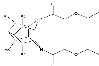
Рис. Структурная формула новой молекулы (этовюрцин)
