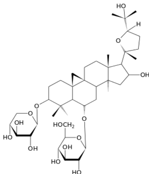
Рис 1. Структура циклосиверсиозида F
