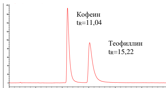
Рис. 3. Хроматограмма смеси кофеина ( k'_{\text{кофеин}} = 3,42 ) и теofilлина ( k'_{\text{теofilлин}} = 5,09 ) при работе на фенильной стационарной фазе с подвижной фазой этилацетат – буфер триэтиламмония ацетата 20 мМ (99,9:0,1), подкисленный уксусной кислотой (40 мМ). Длина волны детектирования: \lambda = 275 нм; Температура термостата колонки: 30 °С; Объем вводимой пробы: 50 мкл. Объемная скорость потока: 1,0 мл/мин.
