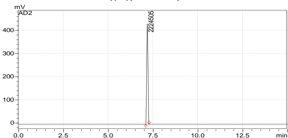
Рис. 2. Метод ВЭЖХ (ELSD) для стандарта циклосиверсиозида F (0.45 mg / mL)
