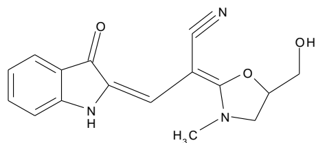
Рис. 1. Структурная формула GRS
