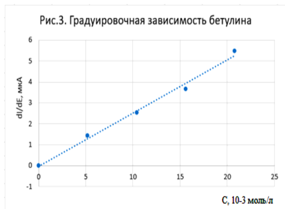
Рис. 3. Градуировочная зависимость бетулина, полученная на графитовом электроде. Фоновый электролит – 0,1М раствор натрия гидроксида.
