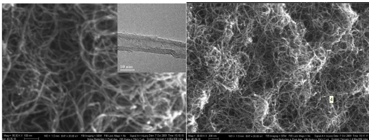
Рис. 1. СЭМ-изображение углеродных нанотрубок «Таунит-М»
