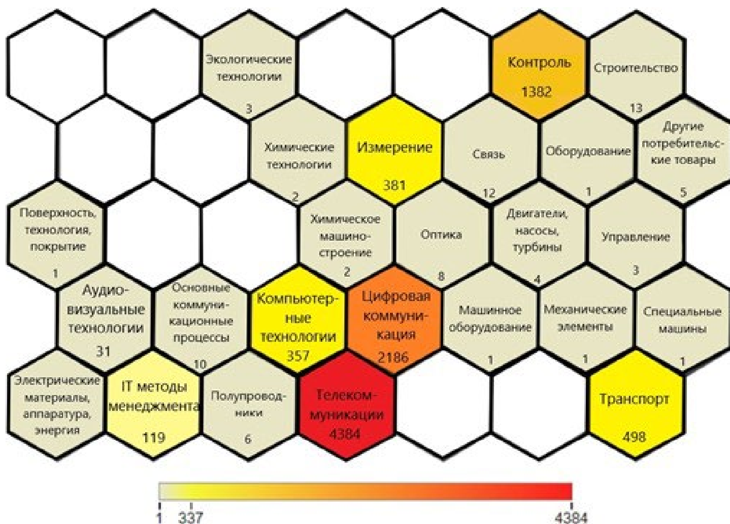
Рисунок 6 – Технологические сегменты
